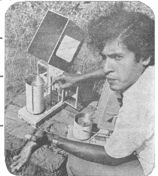
මනා ජල පාලනයක් සඳහා උවමනා වන උපකරණ කිහිපයක් වෙල්යාය මැද සවිකර ඇත. (වමේ) සන්දින වර්ෂාපතන මාපකය, (මැද) දෛනික වර්ෂාපතන මාපකය, (මැද ඇතින්) වැස්සක් පිළිබඳව කල්තබා අඟවන ආර්ද්‍රතා මාපකයක් ද සහිත සුළඟේ වේගය දක්වන උපකරණය, (මැදළහින්) දෛනික ජල වෘෂ්ඨි භවනය සටහන් වන උපකරණය
