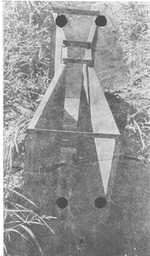
මනා ජල පාලනයක් සඳහා උවමනා වන උපකරණ කිහිපයක් වෙල්යාය මැද සවිකර ඇත. (වමේ) සන්දින වර්ෂාපතන මාපකය, (මැද) දෛනික වර්ෂාපතන මාපකය, (මැද ඇතින්) වැස්සක් පිළිබඳව කල්තබා අඟවන ආර්ද්‍රතා මාපකයක් ද සහිත සුළඟේ වේගය දක්වන උපකරණය, (මැදළහින්) දෛනික ජල වෘෂ්ඨි භවනය සටහන් වන උපකරණය
